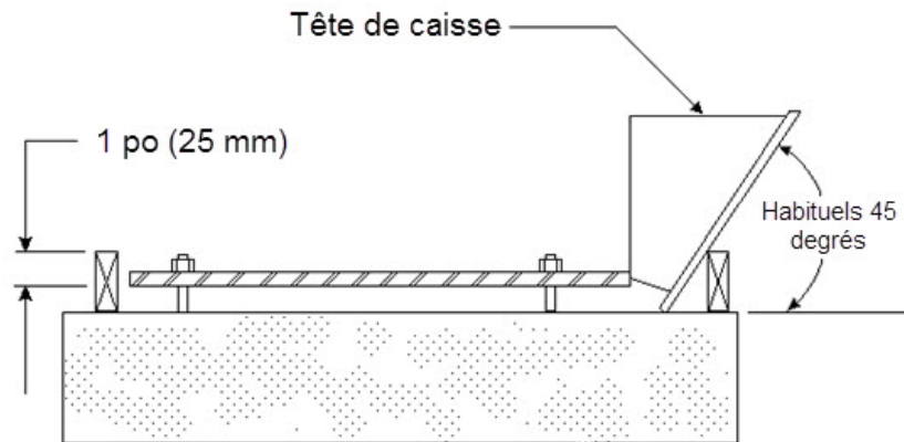
Coffrage avec tête de caisse
