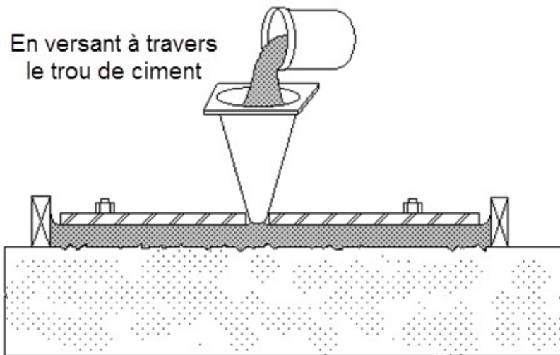
Coffrage avec tête de caisse
