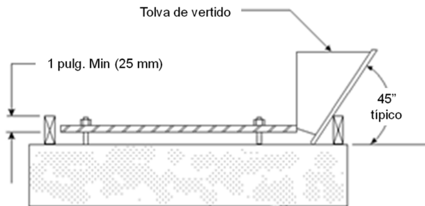
Encofrado con cajón/tolva de vaciado
